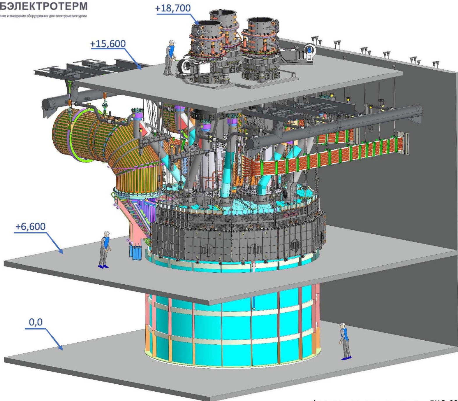
Ферросплавная электропечь РКО-23 (Печь №45, 23 МВА), для производства ферросиликомарганца, цех №7 АО «ЧЭМК». 22.03.2022 г.
